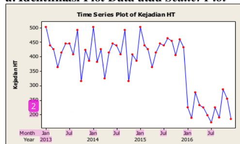
Gambar 3 Plot Data Bulanan Kejadian Hipertensi di Puskesmas Bareng Tahun 2013-2016
