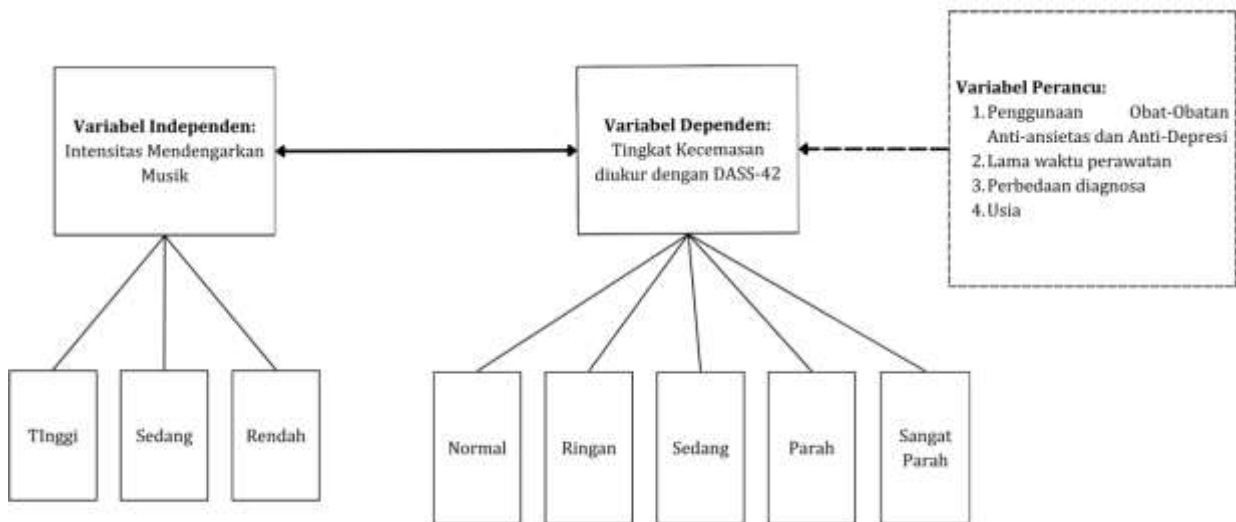
Gambar 3.1 Kerangka Konsep
